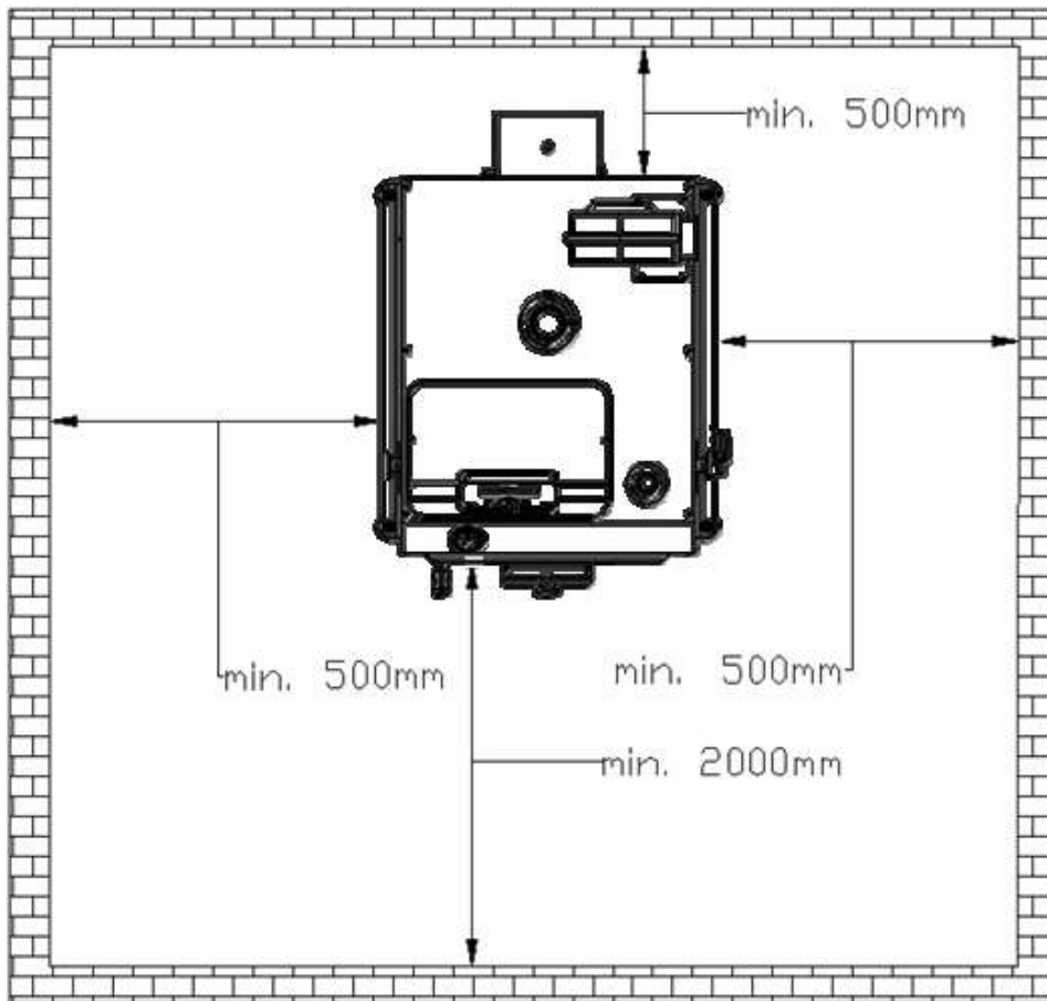
Rys. 3. Ustawienie kotła Kamen w pomieszczeniu kotłowni.
