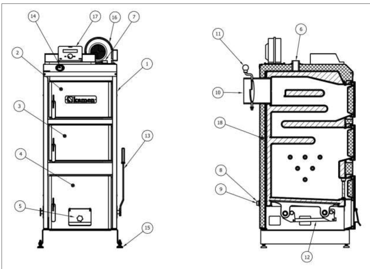
Rys 1. Schemat kotła Kamen WG Premium Agro (podstawowe elementy kotła + przekrój).
