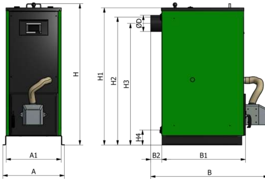
Rys. 2. Podstawowe wymiary kotła Kamen PERFECT Bio.
