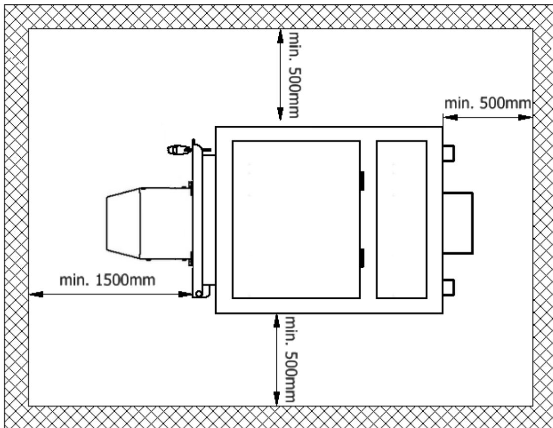
Rys. 3. Ustawienie kotła Kamen w pomieszczeniu kotłowni.
