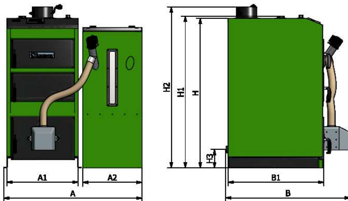
Rys. 2. Podstawowe wymiary kotła Kamen PELLET Kompakt.
