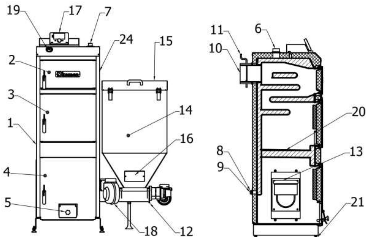
Rys 1. Schemat kotła Kamen MULTI plus Agro (podstawowe elementy kotła + przekrój).
