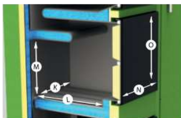
Rys. 2. Podstawowe wymiary kotła Kamen MULTI plus Agro.
